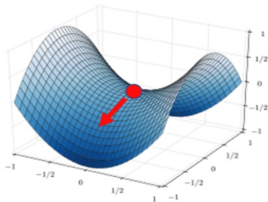
鞍点
