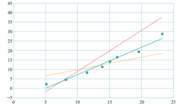
图 4.1 火灾影响的森林面积与气温之间的关系
