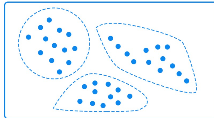
聚类
